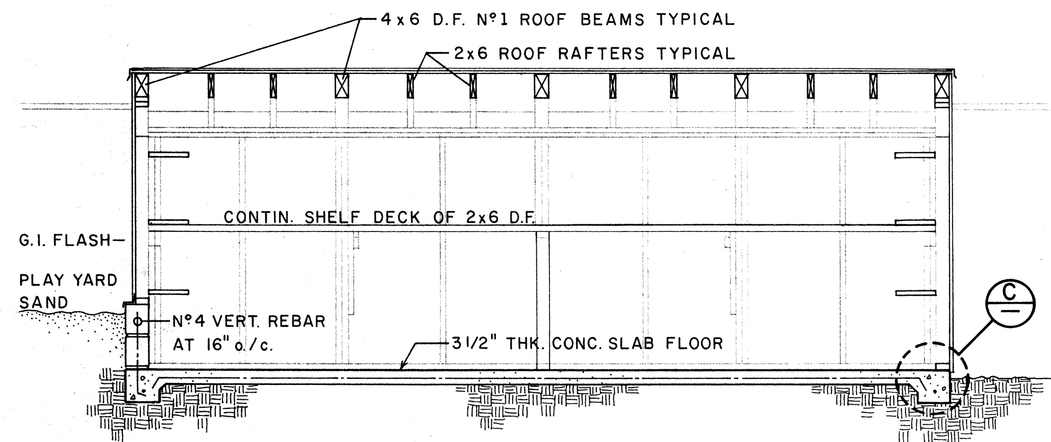
LONGITUDINAL SECTION
